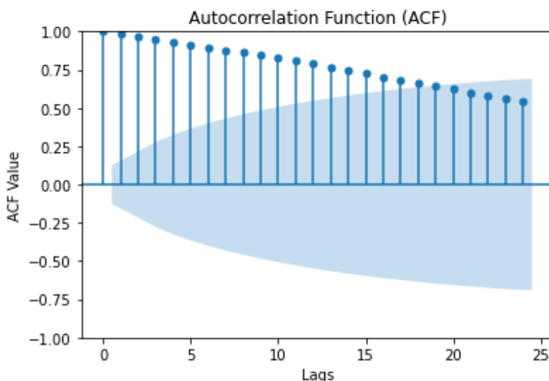
Figura 7 - Função de Autocorrelação (ACF) da variável diferimento - dados mensais
