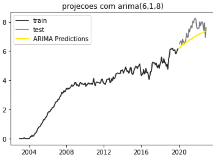
Figura 11 - Projeções com ARIMA (6,1,8)
