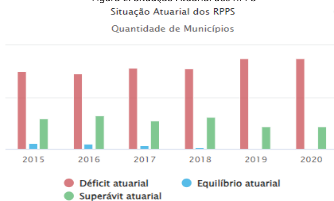
Figura 2: Situação Atuarial dos RPPS
