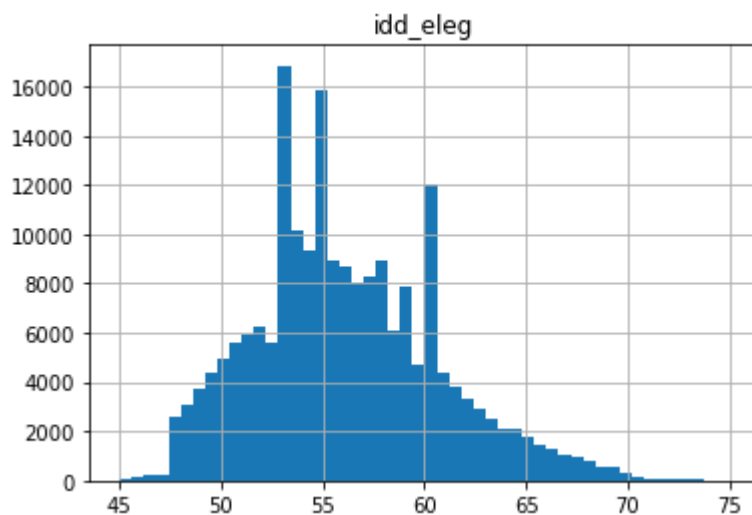
Figura 1 - Histogramas de frequências - amostra geral - Idade Elegível
